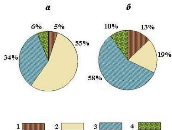
Рис. 95. Химический (групповой) состав торфа верхового типа: а – степень разложения 10 %; б – 55 %. 1 – битумы, растворимые в бензоле; 2 – вещества углеводного комплекса (водорастворимые, легкогидролизующие, целлюлоза); 3 – гуминовые вещества; 4 – негидролизующий остаток
