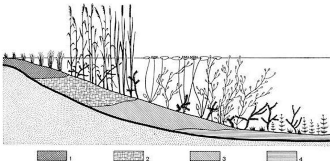
Рис. 8. Схема зарастания озера. Растительность (начиная от берега): осоки, тростник, камыш и рогоз (с примесью погруженных в воду растений); кувшинки; кубышки и другие растения с плавающими листьями; рдесты и другие погруженные в воду растения; донные мхи и водоросли (глубоководная часть озера без высших растений), 1 – осоковый торф; 2 – тростниковый и камышовый торф; 3 – сапропелевый торф; 4 – сапропели (Сукачёв В.Н., 1926)
