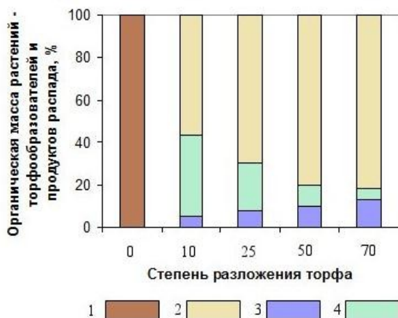
Рис. 94. Динамика процесса распада органической массы растений верхового типа: 1 – органическая масса растений торфообразователей; 2 – потери органического вещества при образовании торфа; 3 – продукты распада; 4 – остатки растительного волокна в торфе
