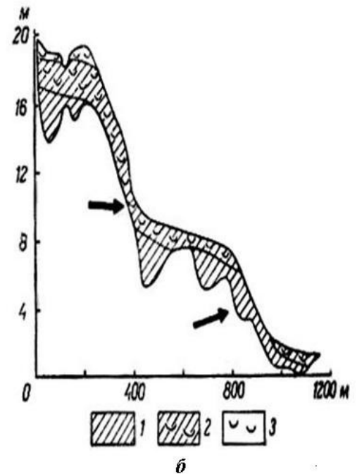
Рис. 83. Висячее болото (а) и его стратиграфический разрез (б) (Г.Е. Елина, 1987): 1 – низинный торф, 2 – переходный, 3 – верховой. Стрелками показано направление поступления напорных грунтовых вод
