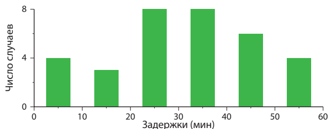
Рис. 4. Распределение задержек Pc1 по длительности при западном дрейфе по данным наблюдений в Борке и Мондах.
