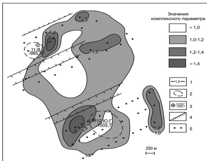
Рис. 5. Карта распределения комплексного параметра в приповерхностных отложениях Вольновской площади. Условные обозначения: 1 – изолинии комплексного параметра. Прочие обозначения см. рис. 4.
