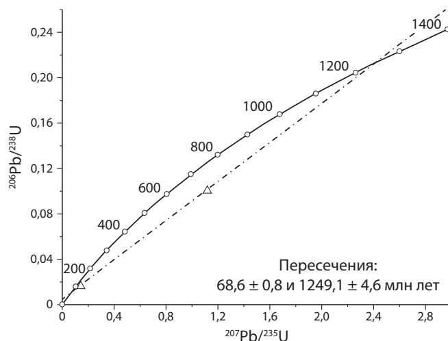
Рис. 4. Диаграмма с конкордией для образца К-Т. Треугольники – наблюдаемые значения изотопных отношений. Пунктирная линия – дискордия.
