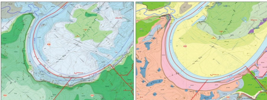
Рис. 6. Фрагменты геологических карт. На карте дочетвертичных отложений (слева) основной фон на большей части территории представлен отложениями юрской (J, голубые оттенки) и меловой (K, зелёные оттенки) систем. На карте четвертичных отложений (справа) полосой по правому крутому борту долины р. Москва протягивается контур делювия (отложения оползней) верхнечетвертичного-голоценового возраста (розовый цвет) [7].
