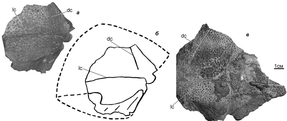
Рис. 3. Передние спинно-боковые кости (anterior dorso-lateralia) Livosteus aff. L. grandis (Gross): а – правая, экз. МЗ МГУ № 134/9, снаружи; б – предполагаемая реконструкция этого экз. снаружи; в – левая, экз. МЗ МГУ № 134/10, снаружи. Средний девон, живет, ардаатовский горизонт Павловского карьера, Воронежская область. Условные обозначения см. в тексте.
