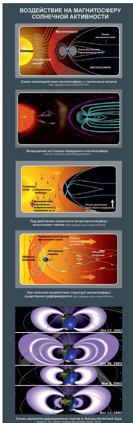
Рис. 4. Воздействие на магнитосферу солнечной активности.
