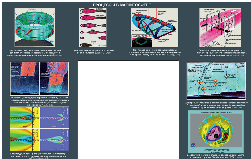
Рис. 3. Процессы в магнитосфере. Fig. 3. Processes in the magnetosphere.
