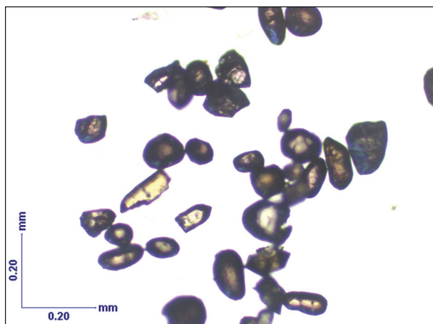
Рис. 3. Сиреневые цирконы, имеющие округлую или овальную форму, из образца К-Т. Fig. 3. Lilac rounded or oval-shaped zircons from the K-T sample.
