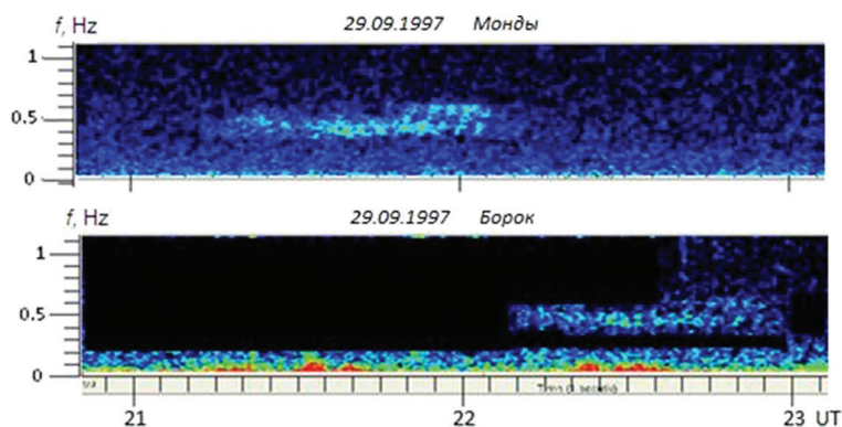
Рис. 2. Пример западного дрейфа серий Pc1. Fig. 2. An example of the western drift of the Pc1 series.
