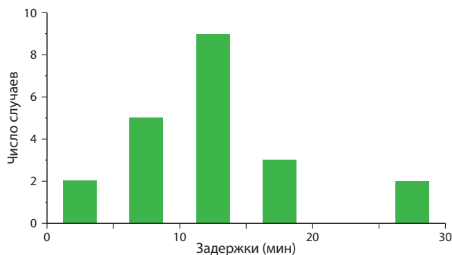
Рис. 7. Распределение задержек Pc1 по длительности при восточном дрейфе по данным наблюдений в Борке и Мондах.
