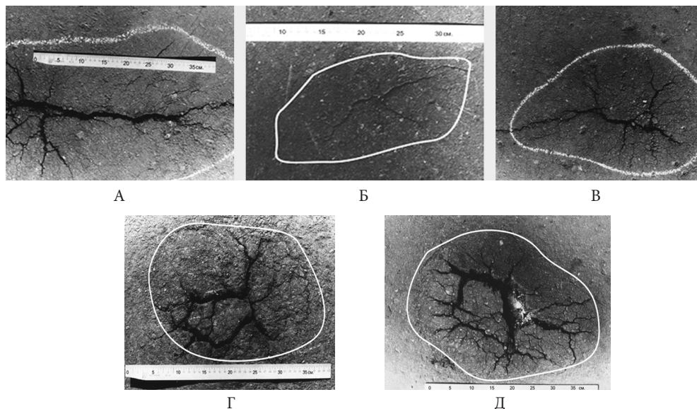
Рис. 1. Результаты натурных наблюдений: А – образование протяжённого линейно вытянутого разрывного нарушения; Б, В – образование линейно вытянутой системы трещин; Г – образование кольцевой системы трещин; Д – система радиальных трещин, осложняющих куполовидную структуру.
