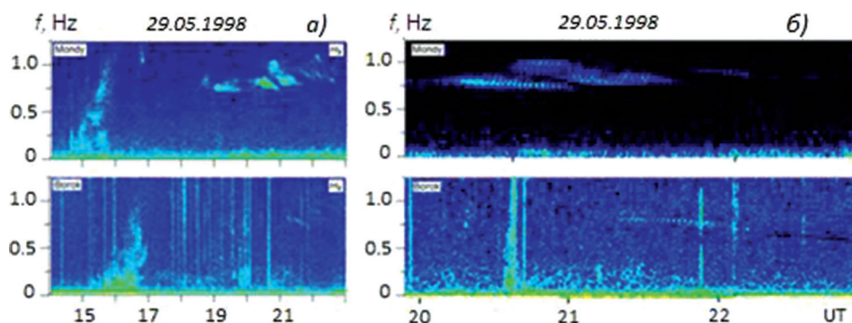
Рис. 8. Западный дрейф пульсаций IpdP и Pc1.
