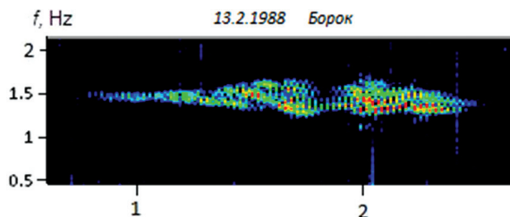
Рис. 1. Динамический спектр серии жемчужин. Здесь и далее UT – Всемирное время, указывается в часах.
