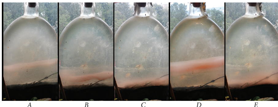
Рис. 2. Вертикальные движения фототрофной бактериальной пластинки (положение фототрофной бактериальной пластинки в разное время суток).
