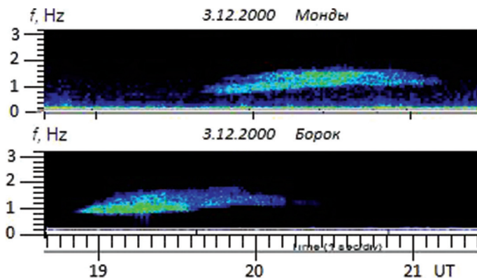
Рис. 5. Пример восточного дрейфа пульсаций Pc1.
