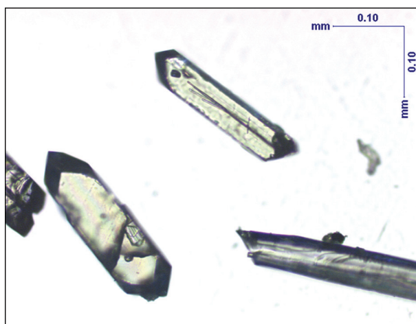
Рис. 1. Бесцветные идиоморфные тонкодлиннопризматические цирконы из образца К-Т. Fig. 1. Colorless euhedral long-prismatic zircons from the K-T sample.
