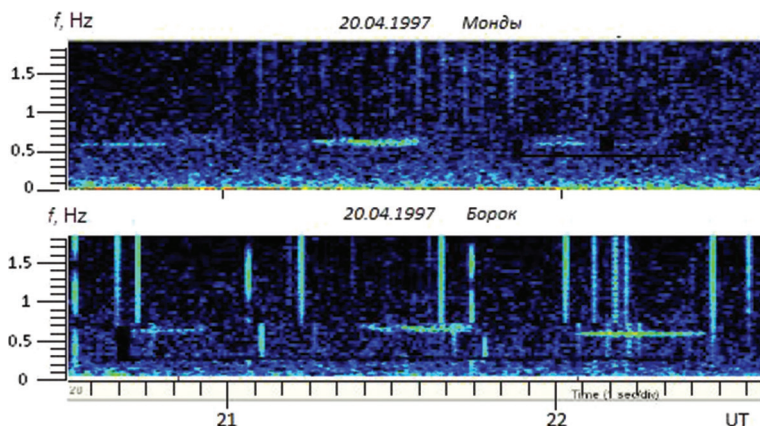
Рис. 3. Проявление эффекта западного дрейфа на примере последовательности из трёх серий Pc1.
