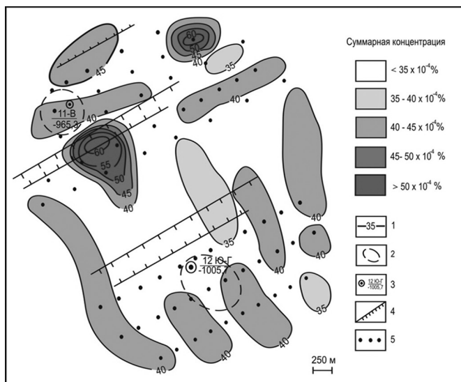
Рис. 4. Карта распределения исходной суммарной концентрации в приповерхностных отложениях Вольновской площади. Условные обозначения: 1 – изолинии суммарной концентрации, 2 – схематическое положение ловушки, 3 – скважины, 4 – граница зоны отсутствия коллекторов, 5 – геоэлектрoхимические пикеты.
