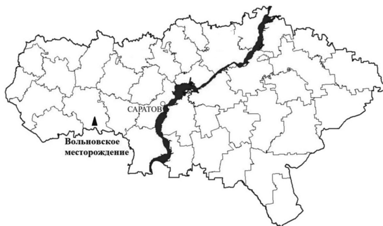
Рис. 2. Схема расположения Вольновского нефтяного месторождения на схеме Саратовской области.
