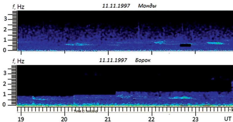
Рис. 6. Эффект восточного дрейфа на примере последовательности из серий Pc1.
