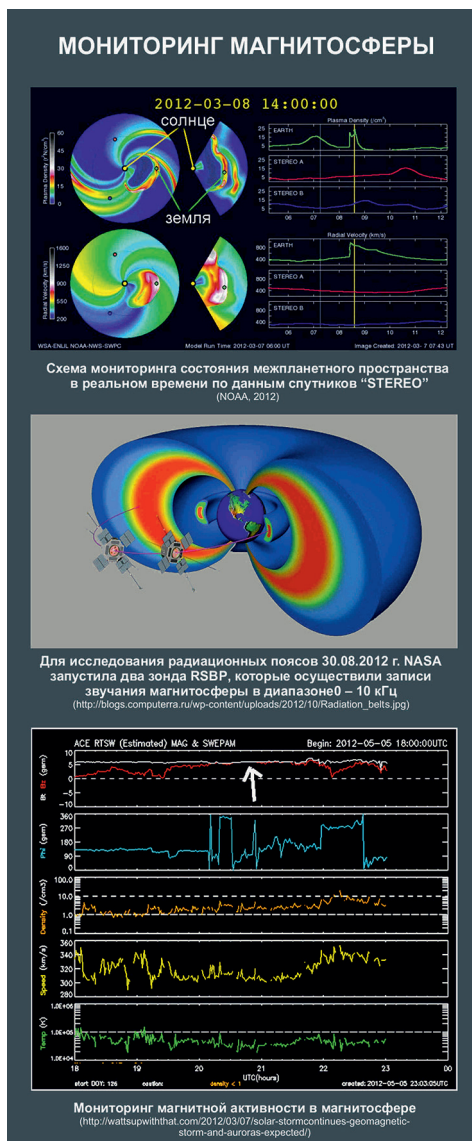
Рис. 6. Мониторинг магнитосферы.
