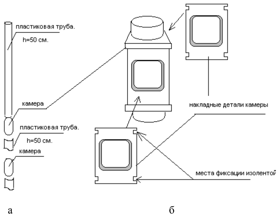
Рис. 27. Собранная конструкция (а); строение камеры (б)
