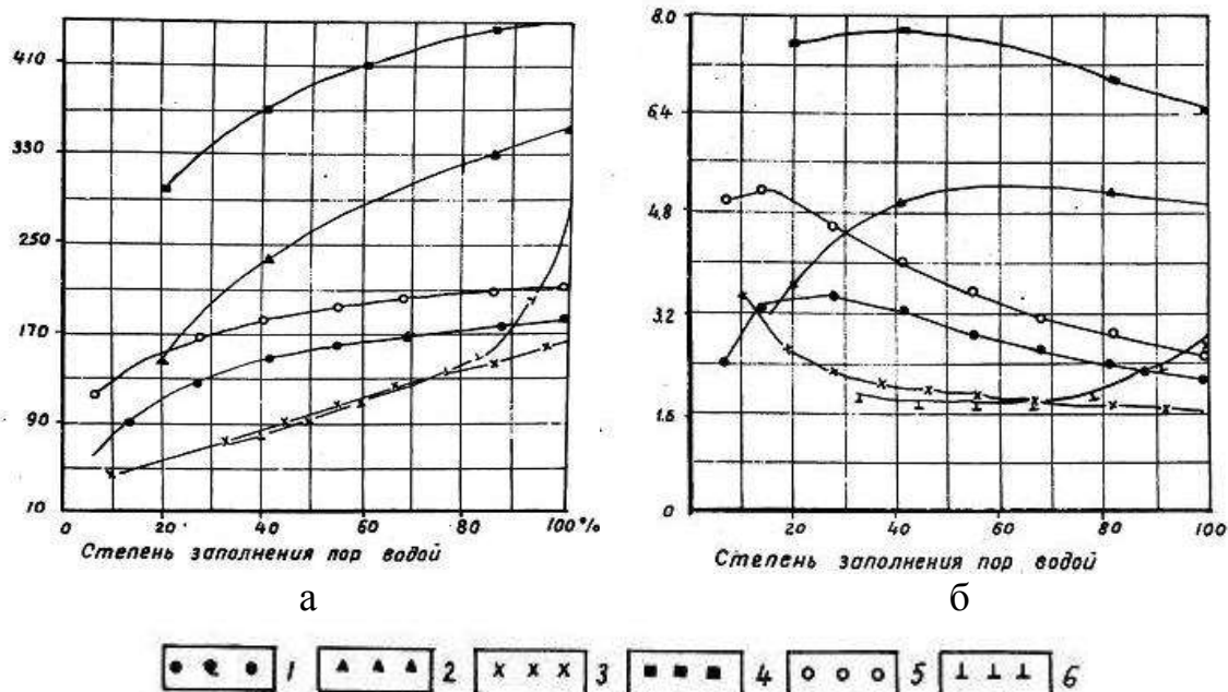
Рис. 14. Тепловые характеристики минеральных и торфяных почв: теплопроводность (а) и температуропроводность (б)
