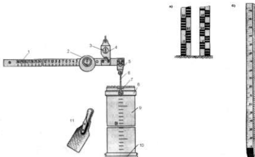
Рис. 7. Снегомер весовой ВС-43 и рейка снегомерная: стационарная (а) и переносная (б)
