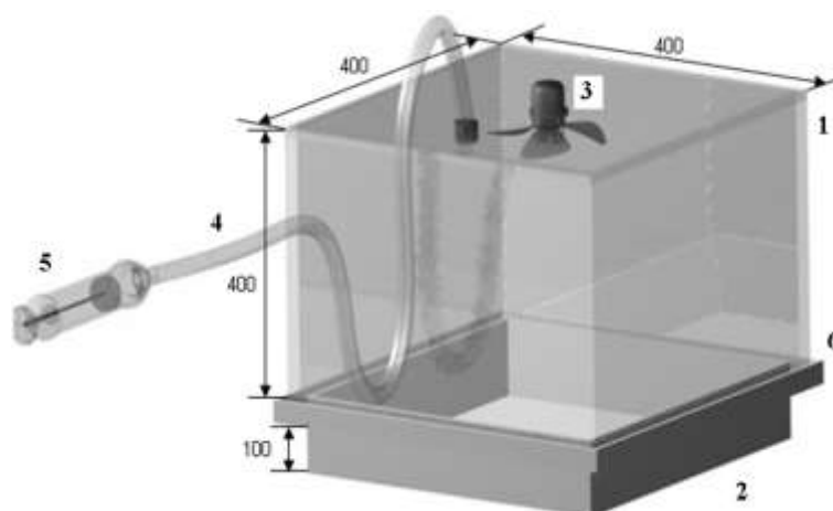
Рис. 38. Камера для измерения эмиссии парниковых газов [17]
